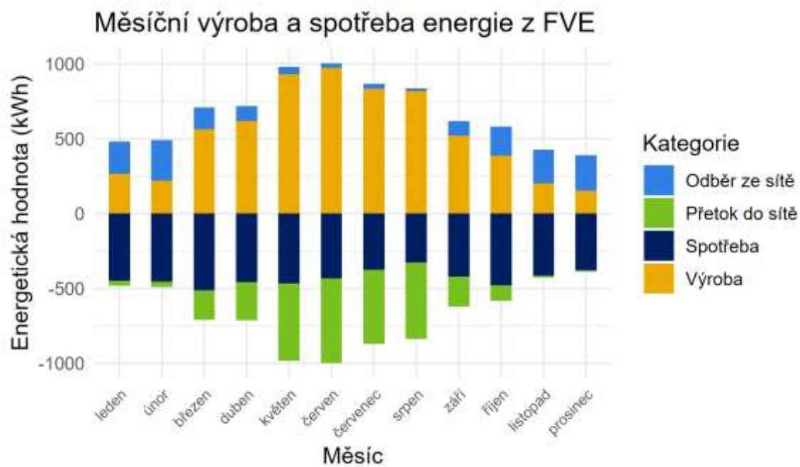
Graf 34: Měsíční energetická bilance pro optimální instalaci – Sportovní areál
