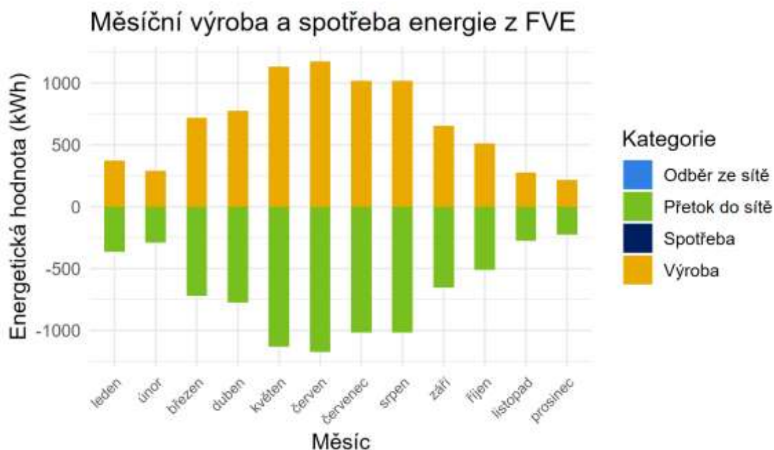
Graf 29: Měsíční energetická bilance pro maximální instalaci – Hostinec obce č.p. 37
