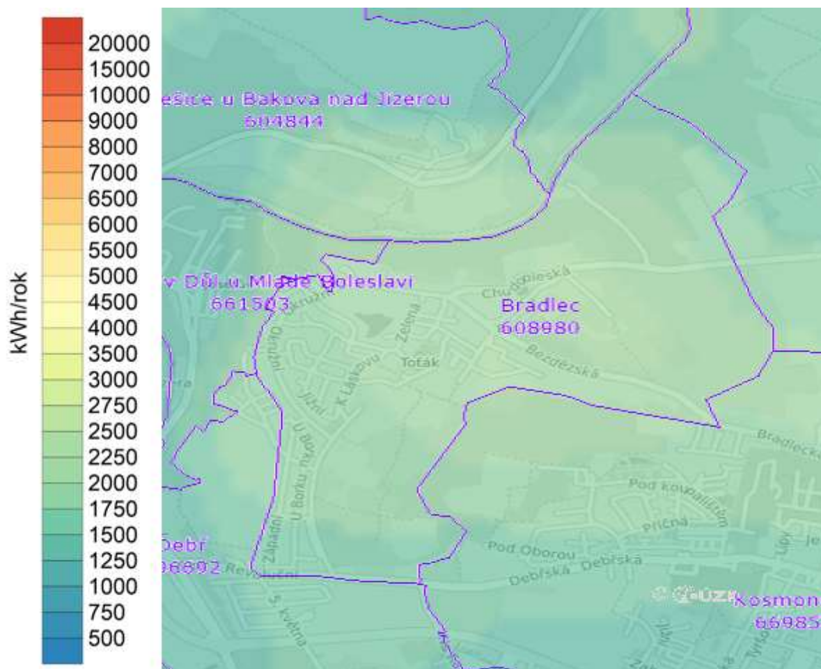
Obrázek 3: Potenciál výroby v obci a jejím okolí
