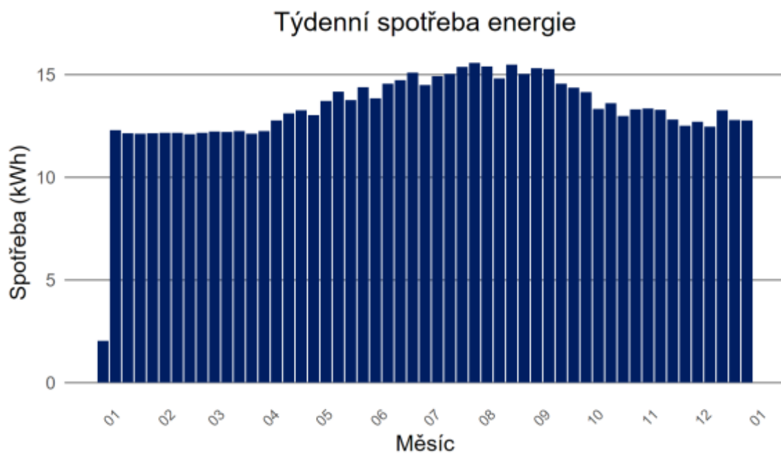
Graf 30: Modelovaná spotřeba objektu po týdnech – Hasiči
