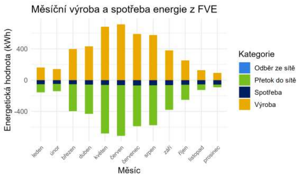
Graf 31: Měsíční energetická bilance pro optimální soběstačnost – Hasiči
