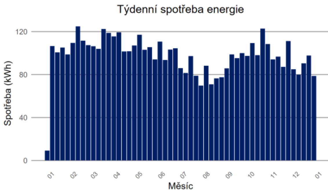
Graf 32: Modelovaná spotřeba objektu po týdnech – Sportovní areál
