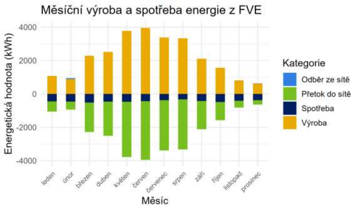
Graf 33: Měsíční energetická bilance pro optimální soběstačnost – Sportovní areál
