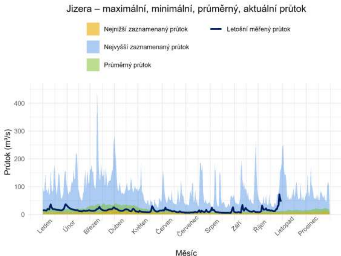
Graf 9: Průběh průtoku – Jizera
